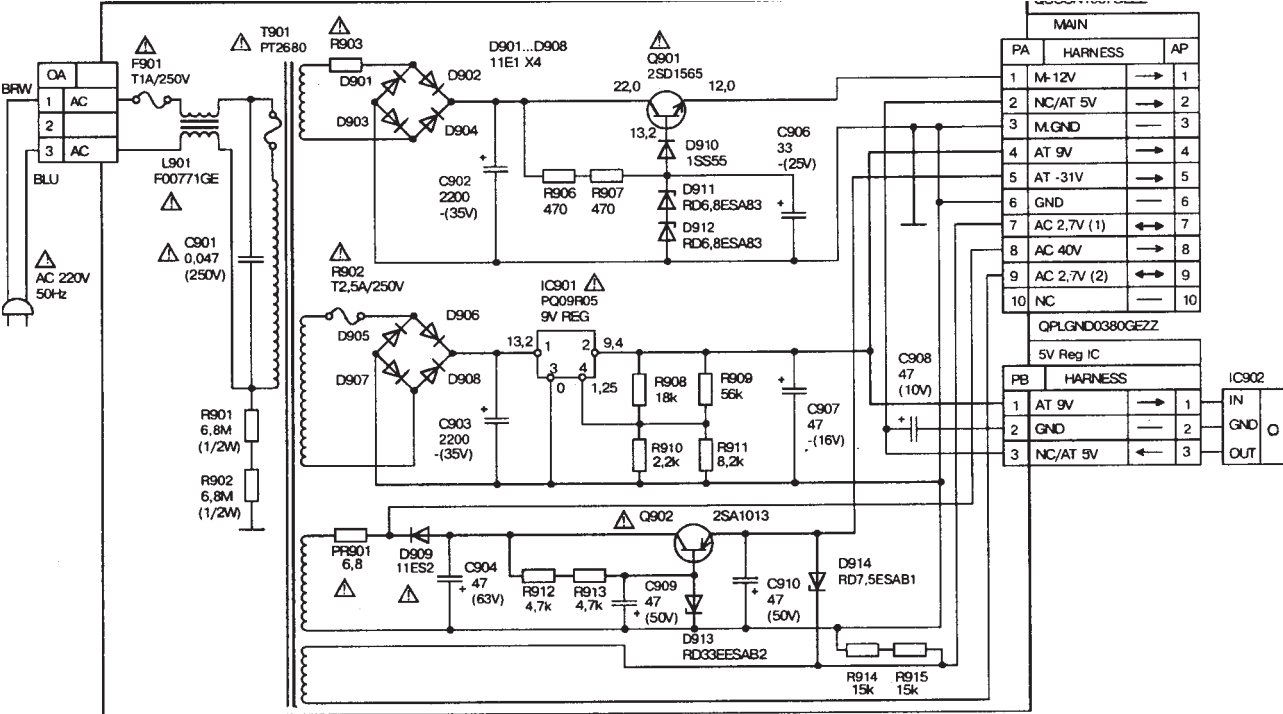
Принципиальная схема источника питания видеомэагнитофона VC-A30B фирмы SHARP.
